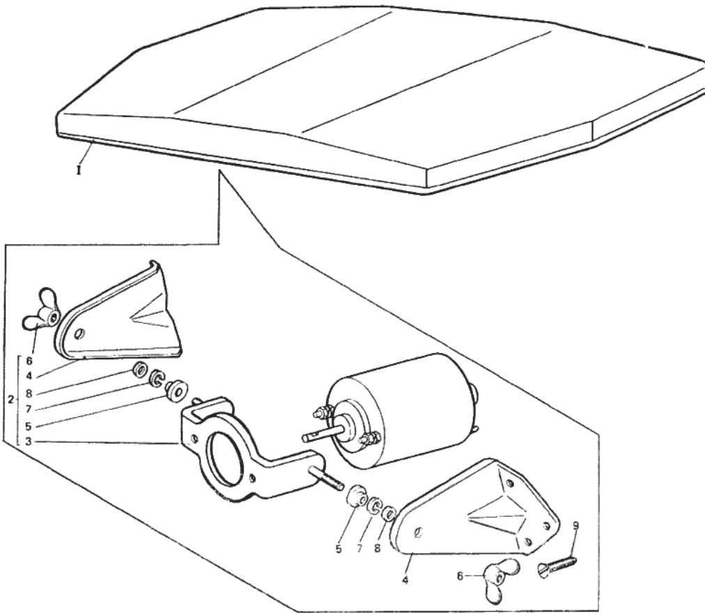
Рис. 147. Крыша кабины Т40М-6707010-А
